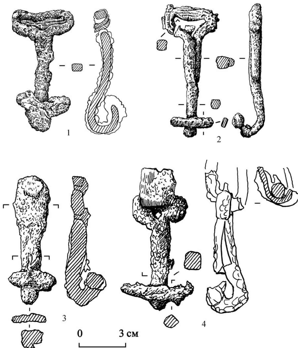
Рис. 1. Колчанные крюки из памятника Яломан II: 1 – курган № 29; 2 – курган № 30; 3 – курган № 31; 4 – курган № 32 (1 – железо с остатками кожи; 2–4 – железо)
