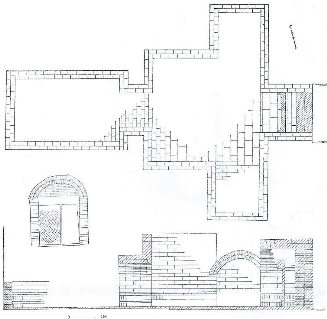
Рис. 2. Конструкция могильного памятника, датированного 8-м годом девиза правления Чжэнши (императора Цао Фана) (по: [Чжан Цзянь, Юй Фувэй, 1989. С. 315])
